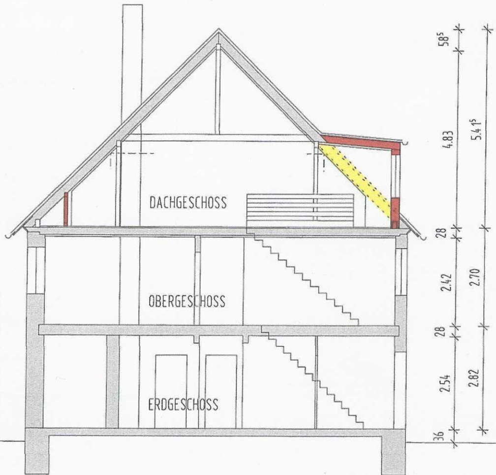
SCHNITT A-A
